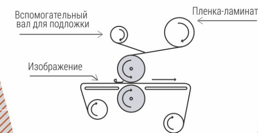
ГОРЯЧЕЕ ЛАМИНИРОВАНИЕ
