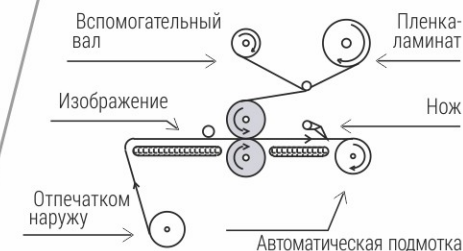
ХОЛОДНОЕ ЛАМИНИРОВАНИЕ
