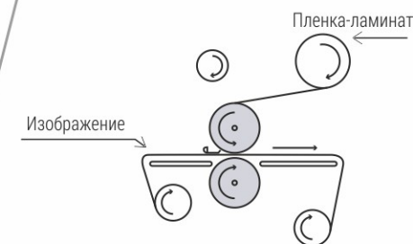
ХОЛОДНОЕ ЛАМИНИРОВАНИЕ
