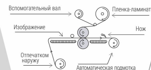
ГОРЯЧЕЕ ЛАМИНИРОВАНИЕ
